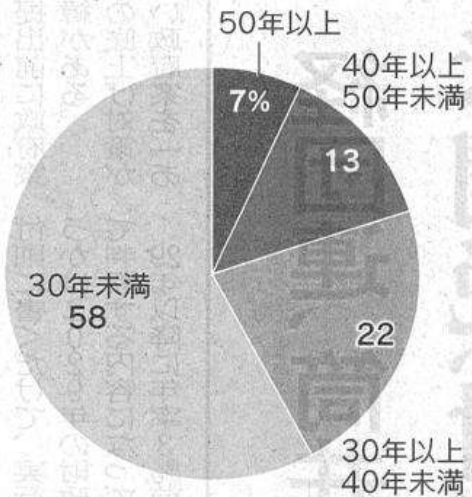
全国の下水道管の老朽化の現状
